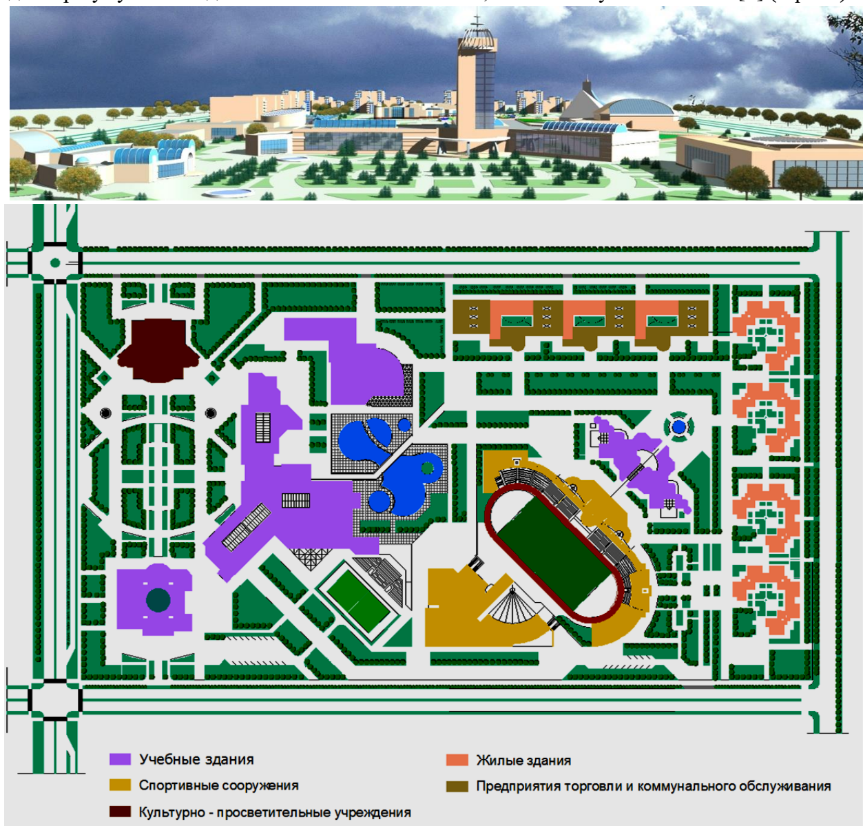
9-расм. Актау шаҳридаги университет мажмуаси лойиҳаси.
